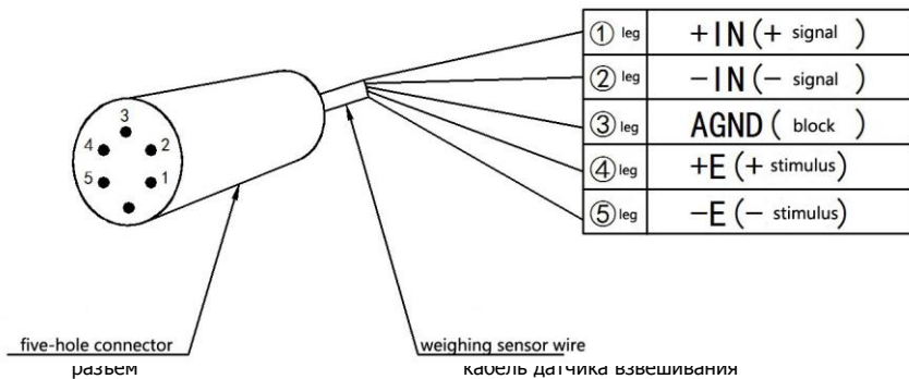
Рисунок 8 (подключение разъема)
